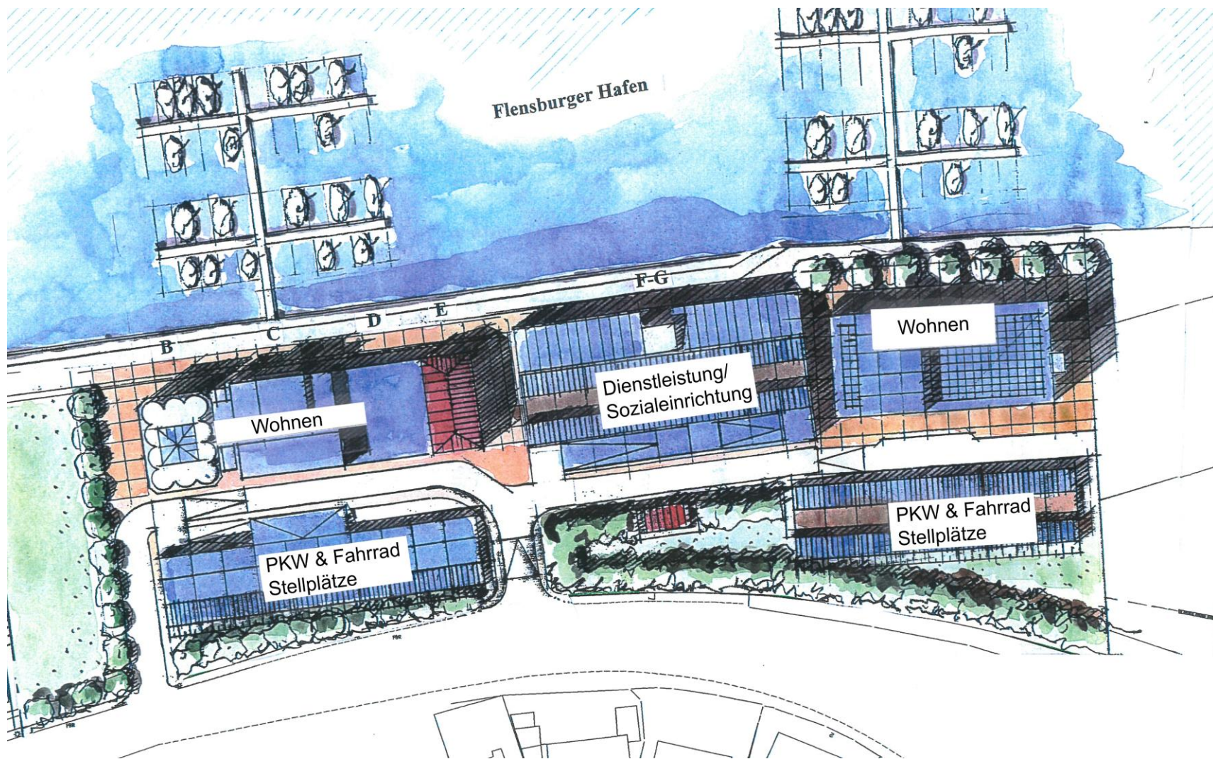
_Lageplan Kaihäuser am Ballastkai
